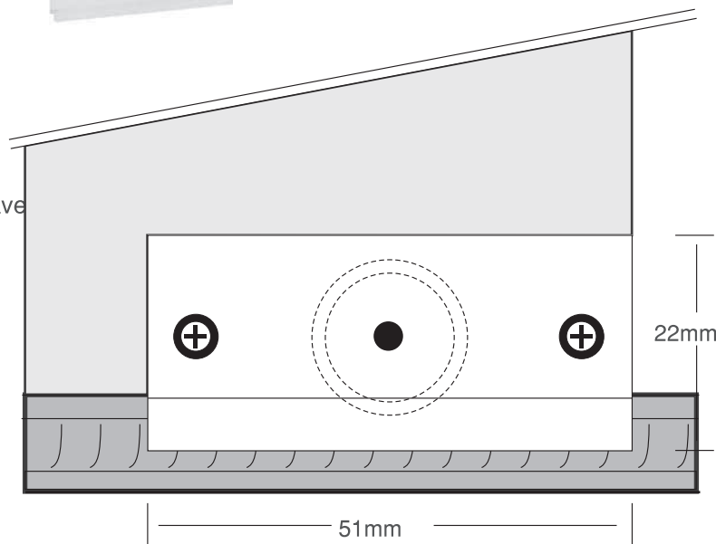
TT419 HEAD GUIDE
