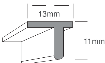
TT419 HEAD GUIDE
